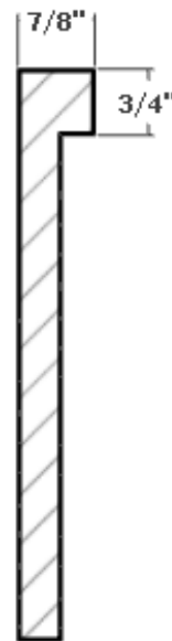
DOOR DETAIL
